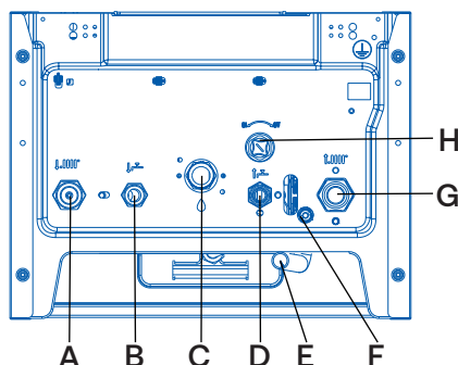
Двухконтурные котлы : EvoLine S 2.24/2.32TW
