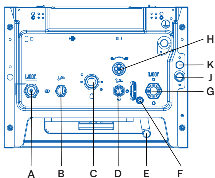
Двухконтурные котлы: GreenLine S 2.35TW
