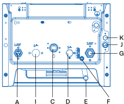
Бір контурлы қазандықтар: GreenLine S 1.35TW
