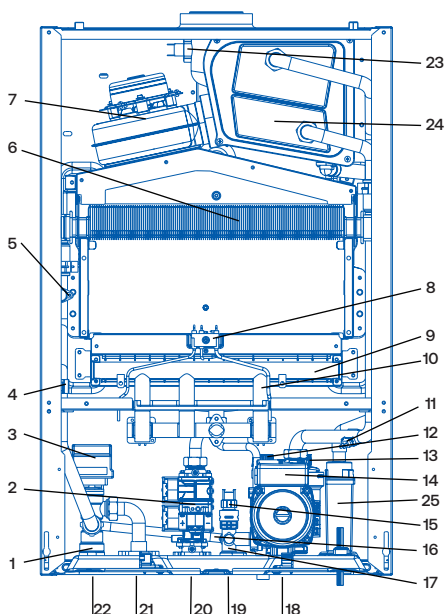
Одноконтурные котлы: GreenLine S 1.35TW
