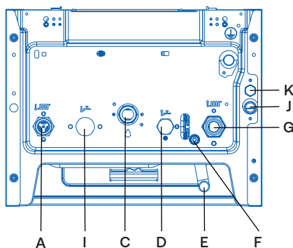
Одноконтурные котлы: GreenLine S 1.35TW
