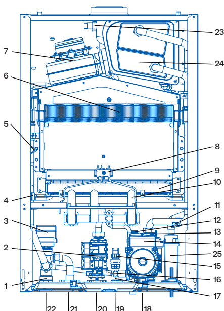
Бір контурлы қазандықтар: GreenLine S 1.35TW
