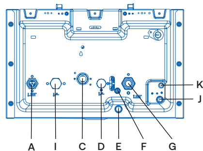
Одноконтурные котлы: GreenLine S 1.35TW
