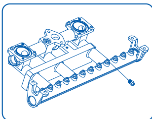
Газовая рампа с форсунками.
