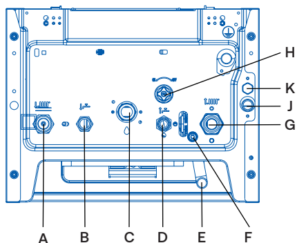
Екі контурлы қазандықтар: GreenLine S 2.35TW
