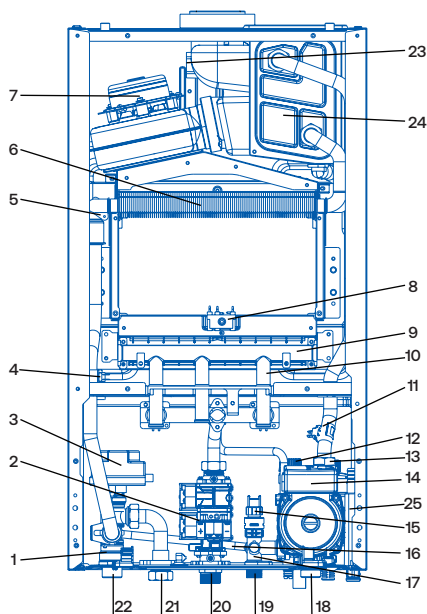
Бір контурлы қазандықтар: GreenLine S 1.20/1.26/1.30TW
