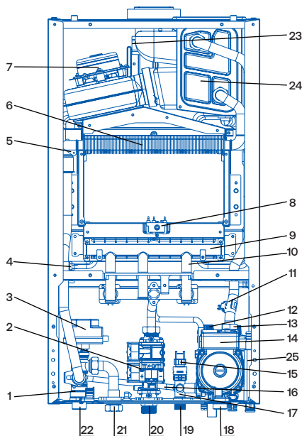
Одноконтурные котлы: GreenLine S 1.20/1.26/1.30TW
